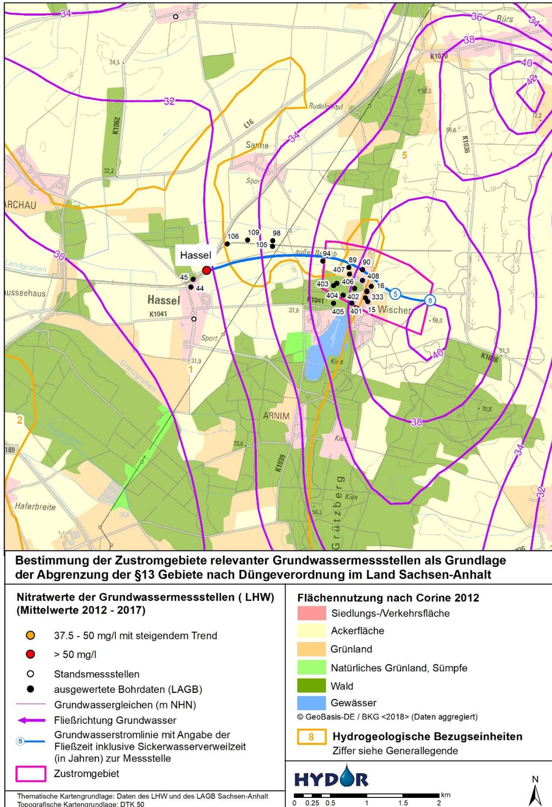
Abb. 10: Darstellung des für die LHW-Messstelle Hassel (mit Überströmung) ausgewiesenen Zustromgebietes mit lithologisch homogener Ausprägung der ungesättigten Zone im Lockergestein
